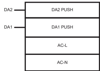
SCHEMA DE CABLAGE DALI
