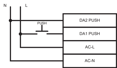
SCHEMA DE CABLAGE BOUTON POUSSOIR
